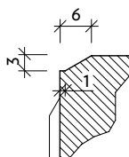
Řez hranou
