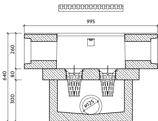
Řez a-a' sestavou
