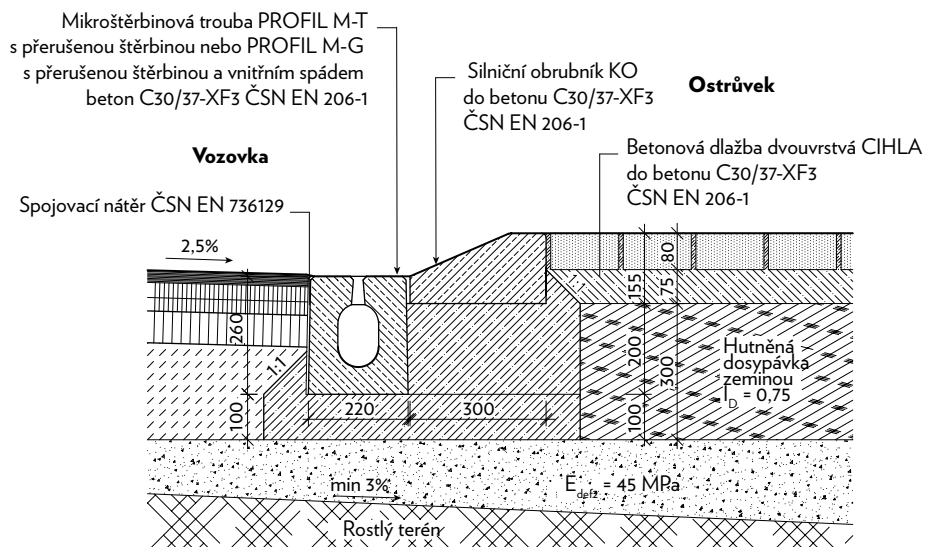
Mikroštěbinová trouba - PROFIL M, vozovka v kombinaci sostrůvkem
