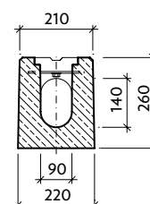
Řez: b-b' M-C0
