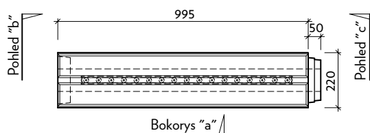
Půdorys
