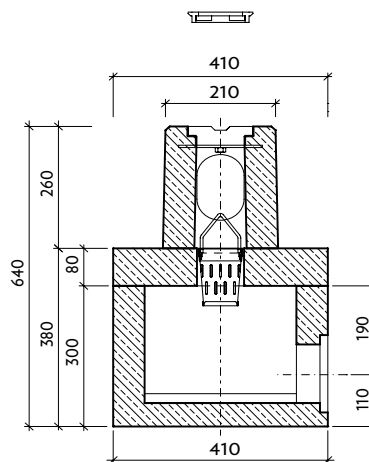
Řez b-b' sestavou
