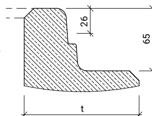
Detail dříku
