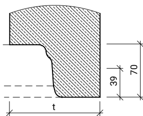
Detail hrdl s těsněním a bez těsnění INTEGRO
