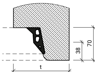
Detail hrdl s těsněním a bez těsnění INTEGRO
