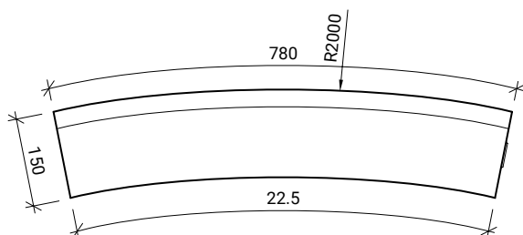
Obrubník silniční H 25 R 2,0
