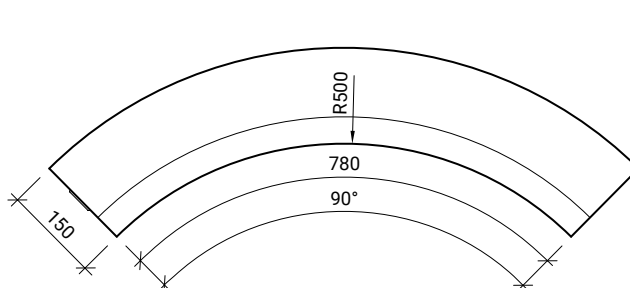
Obrubník silniční H 25 R 0,5
