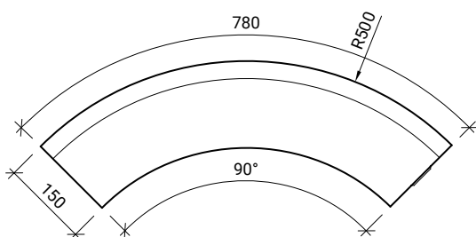
Obrubník silniční H 25 R 0,5
