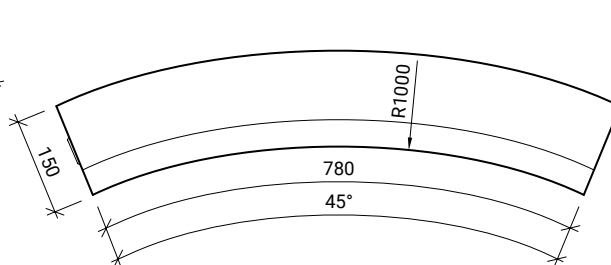
Obrubník silniční H 25 R 1,0
