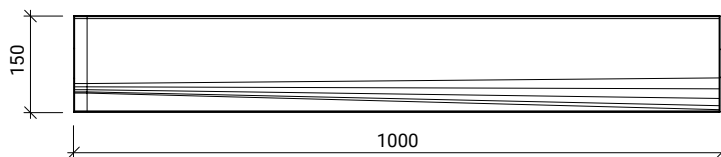
Obrubník náběhový pravý H 25
