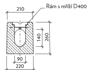
Řez: b-b' M-Co
