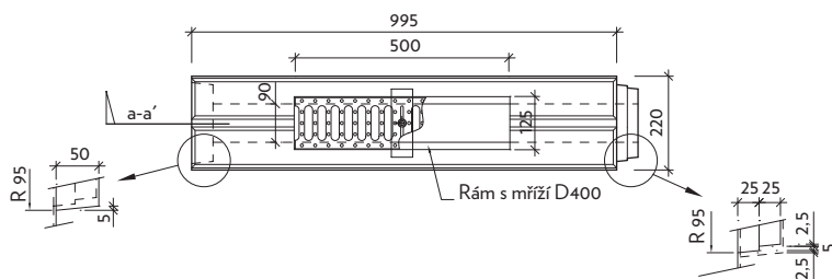
Pohled "a" M-Co - drážka
