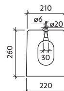
Řez "b-b"
