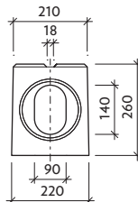
Pohled "b" M-Co - pero
