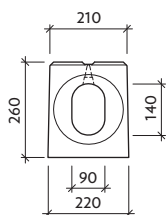
Pohled "b" - drážka
