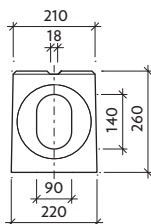
Pohled "a" M-Co - drážka
