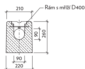
Řez: b-b' M-CS
