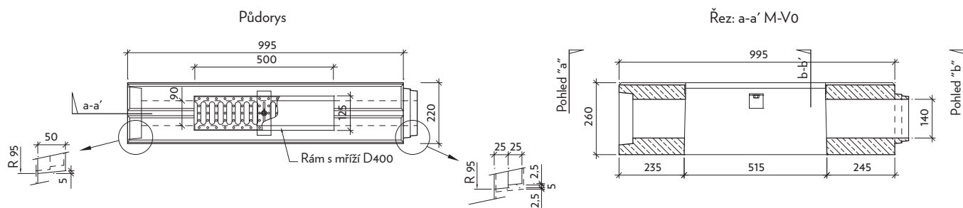
M-V0 – vpusťový kus základní s mříží D400
