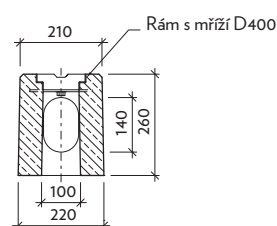
Řez: b-b' M-V0
