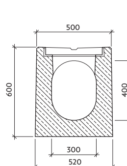
Řez: b-b'
