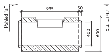
Řez: a-a'
