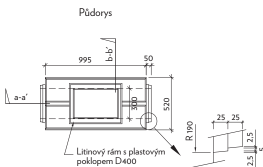
III-1-CS - čistící kus základní s litinovým rámem a plastovým poklopem pro zatížení D400
