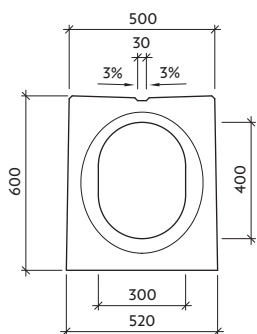
Pohled "a" III-0-V0 - drážka
