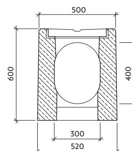
Řez: b-b'
