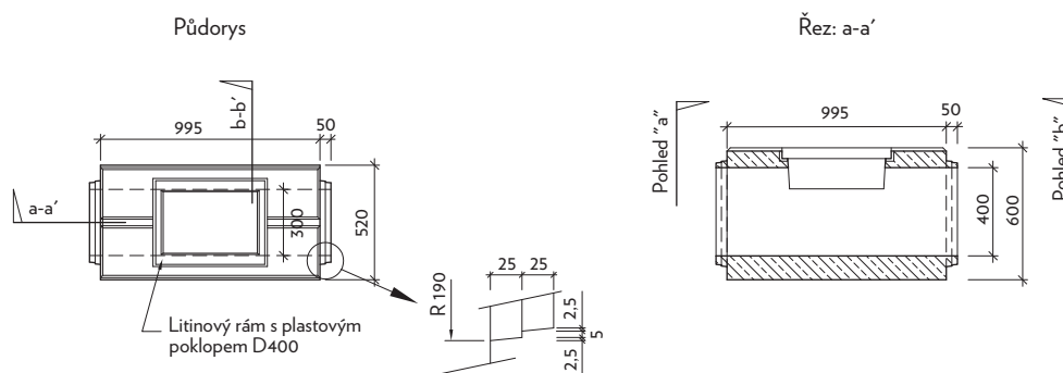
III-0-CS - čistící kus základní s litinovým rámem a plastovým poklopem pro zatížení D400
