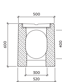
Řez: b-b' III-0-V0
