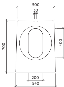
Pohled "a" IV-1-V0 - drážka
