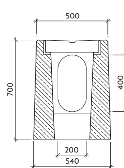
Řez: b-b' IV-1-V0
