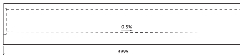
Profil IV-0-G38/40 se spádem dna
