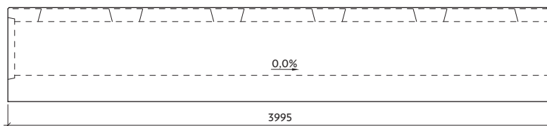
Profil IV-1-T40/40 bez vnitřního pásu
