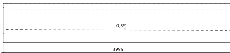
Profil IV-0-G36/38 se spádem dna
