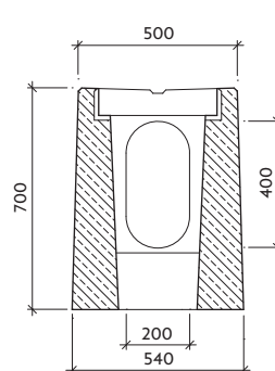
Řez: b-b' IV-1-VU
