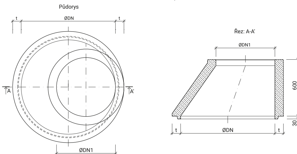
Detail dířku TBR-Q.2
