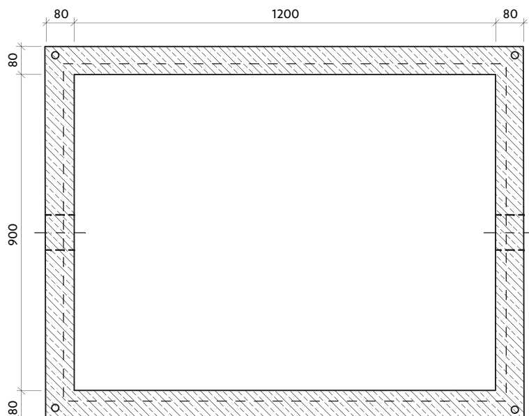
Půdorys
