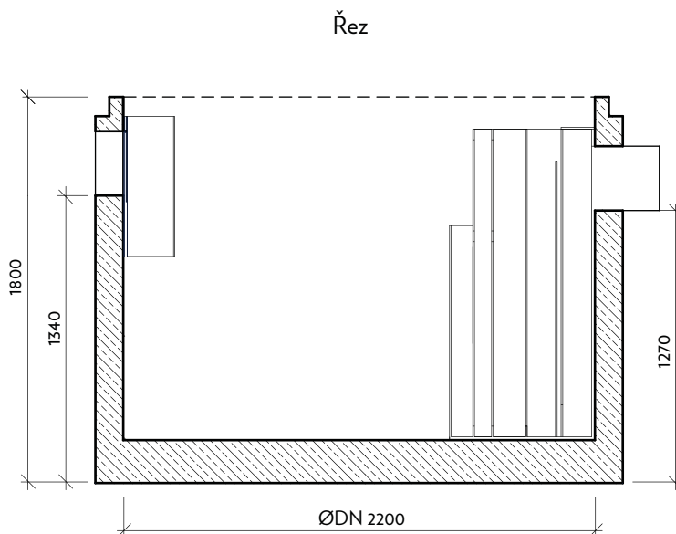
Odlučovač lehkých kapalin
