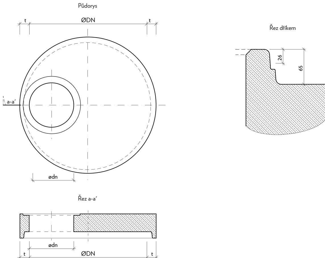
Zákrytová deska
