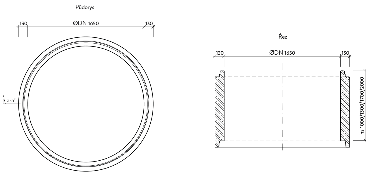
TBZ-Q.1 Jímkové skruže DN 1650
