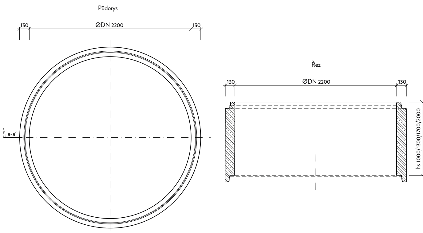
TBZ-Q.1 Jímkové skruže DN 2200
