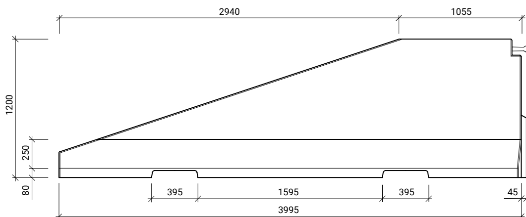
Pohled čelní
