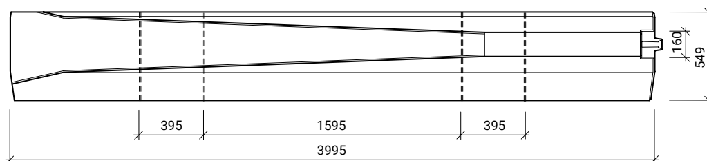
Půdorys
