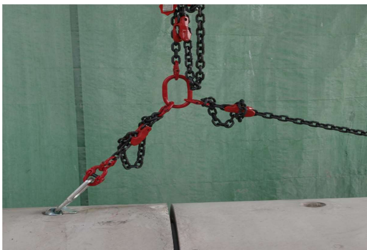
Obrázek č. 9 – Detail řetězového úvazku
