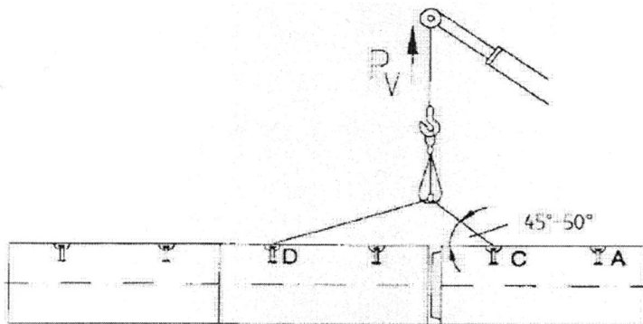
Obrázek č. 8 – Spojování trub pomocí řetězového ukladače
